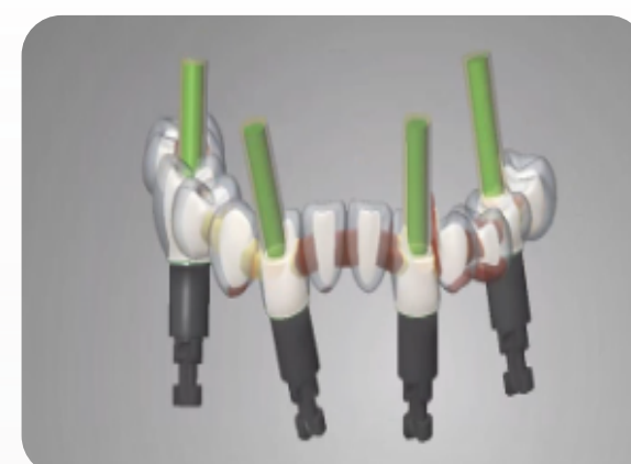
3) Diseño de la barra de dióxido de zirconio en el programa de CAD/CAM.
