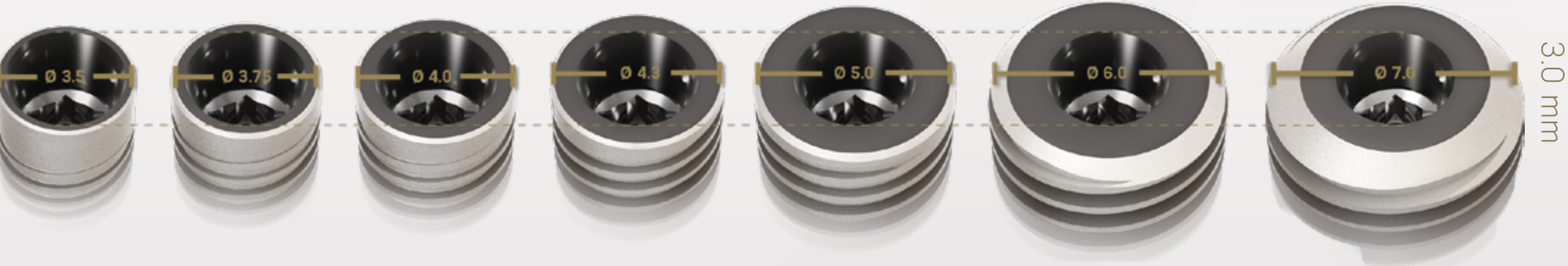
FIGURA 2. Todas las conexiones de implantes Neodent® Grand Morse® tienen las mismas dimensiones, independientemente del diámetro del implante, lo cual se traduce en un proceso protésico más sencillo.
