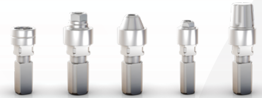
FIGURA 13. Análogos híbridos reposicionables para implante, pilar, Mini pilar cónico, micro pilar y pilar universal Grand Morse®.
